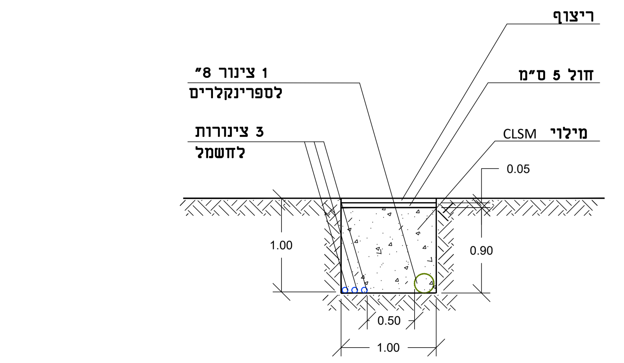
חתך 2-2
