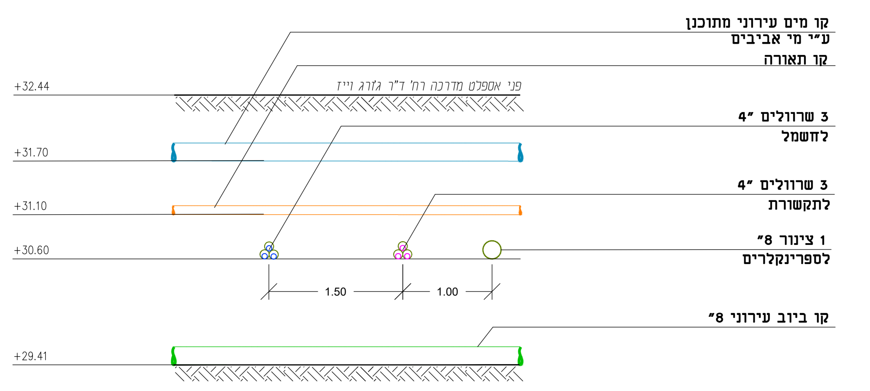
חתך A-A ק"מ 1:50
