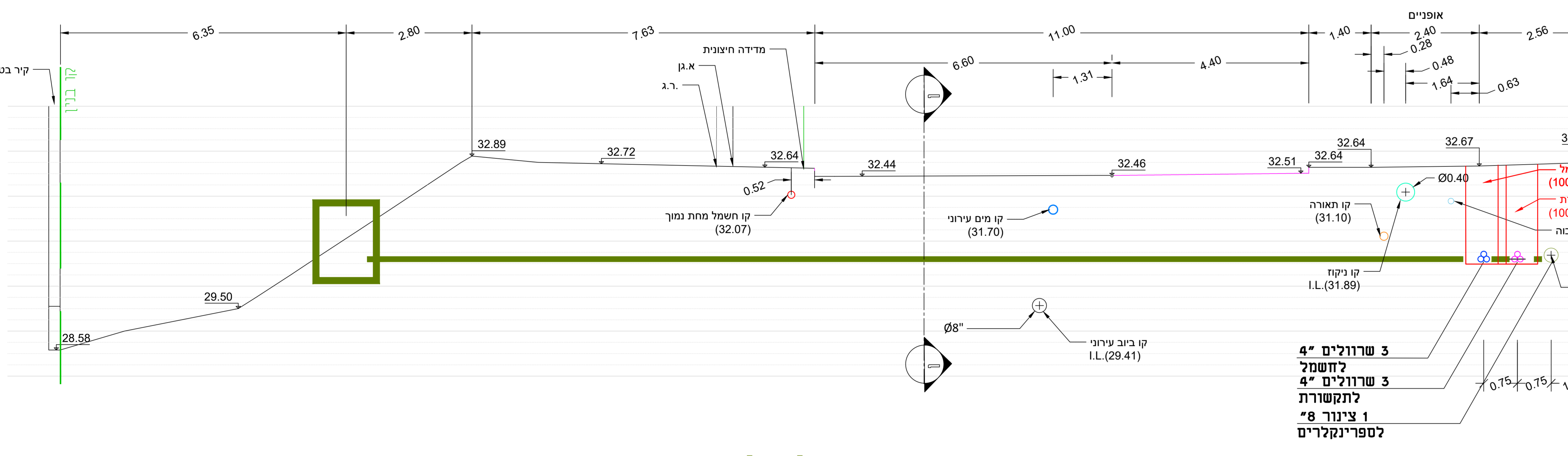
חתך A-A ק"מ 1:50
