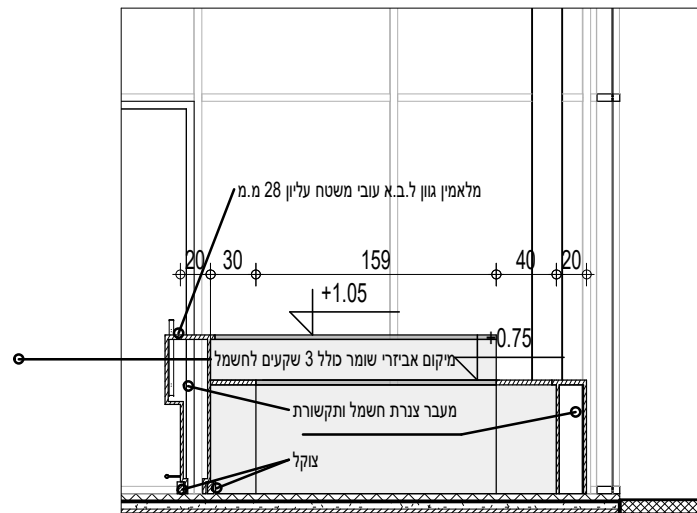
3 חתך 1-1 1 : 50
