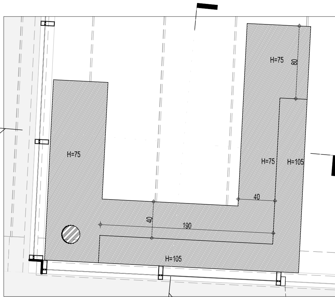
1 תכנית שולחן - מפלס עליון 1 : 25
