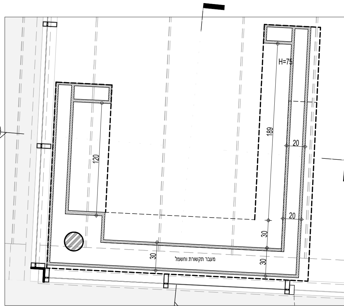
2 תכנית שולחן - מפלס תחתון 1 : 25
