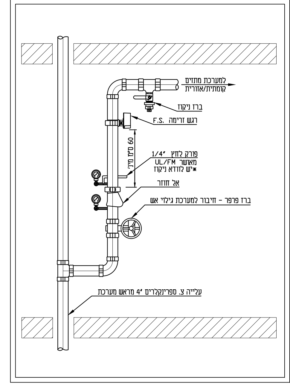
פרט 3 ברז בדיקה וניקוז
