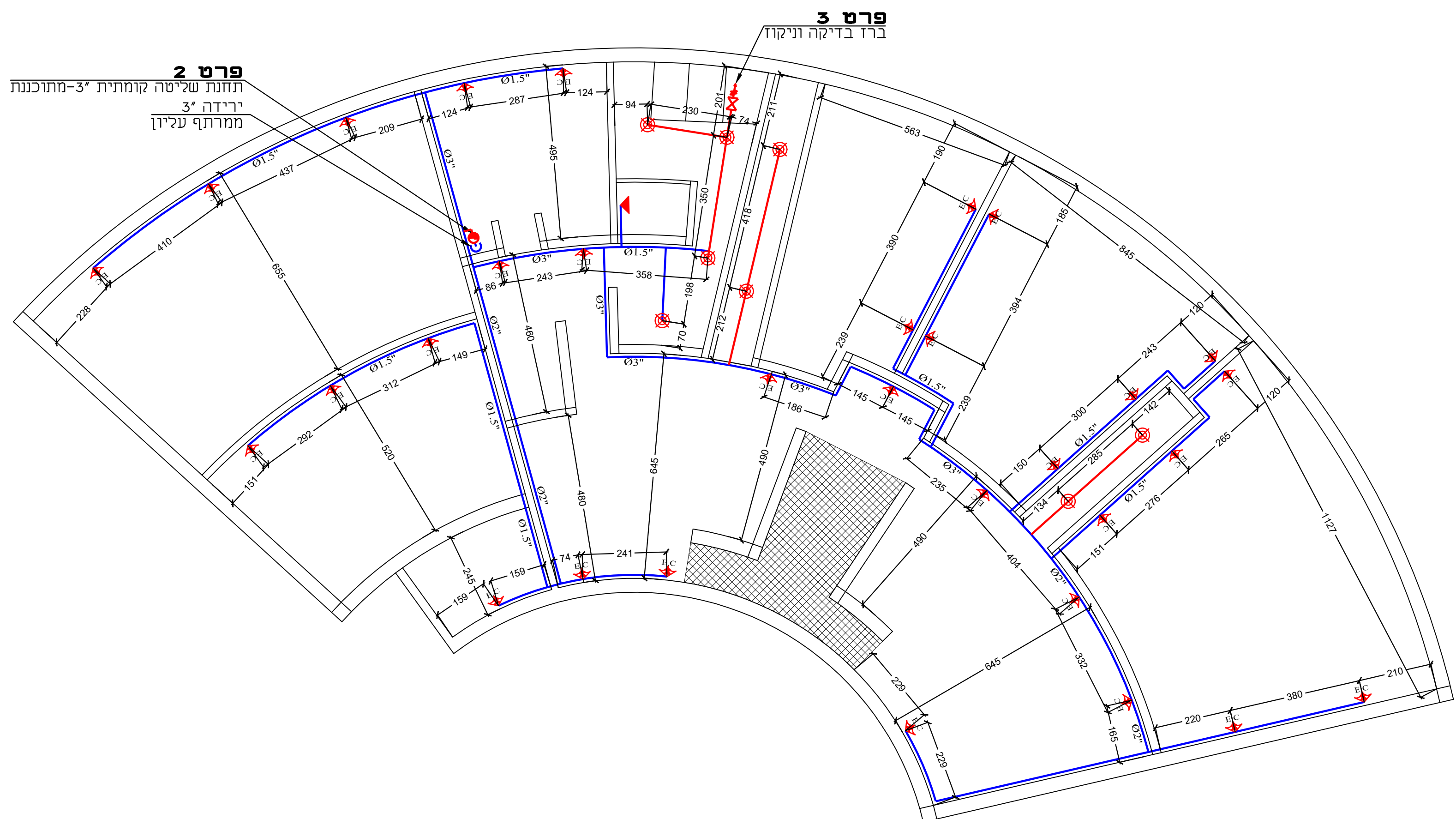
תכנית קומת מרתף תחתון מפלס -6.67
