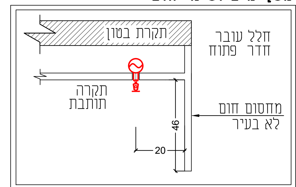
פרט 5 מערכת 0.2" PREACTION DOUBLE INTERLOCK
