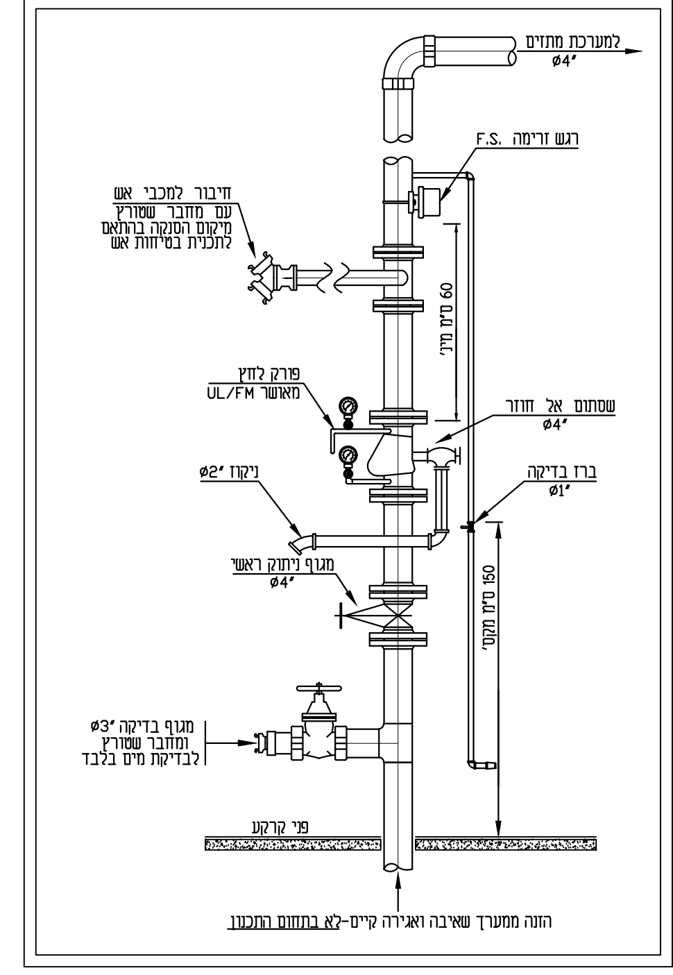
פרט 2 תחנת שליטה קומתית
