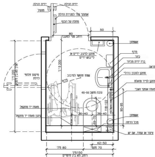
119 – תא בית שימוש נגיש מטיפוס 1, שיש בו אסלה עם מכל הדחה סמוי מחופה לכל רוחב התא
