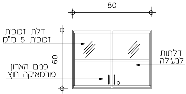
חזית 1:20
