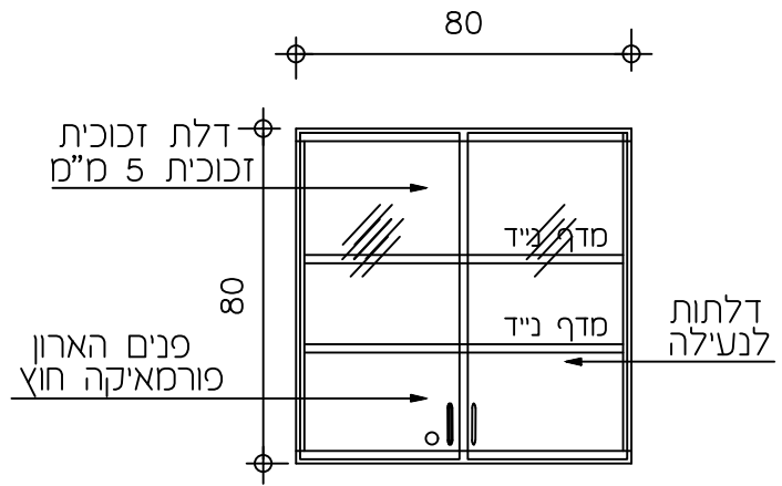
חזית 1:20
