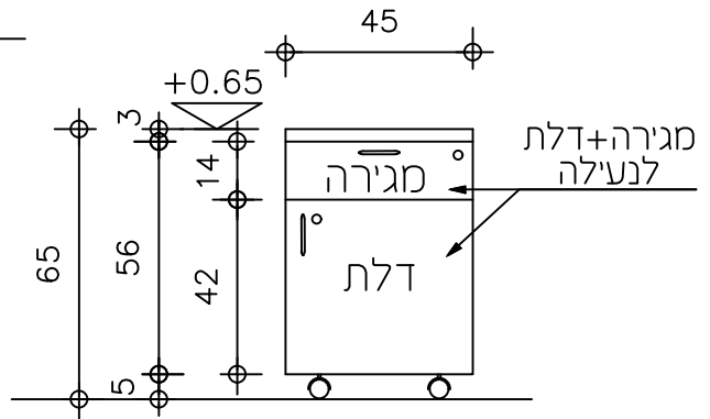
חזית ארונית 1:20
