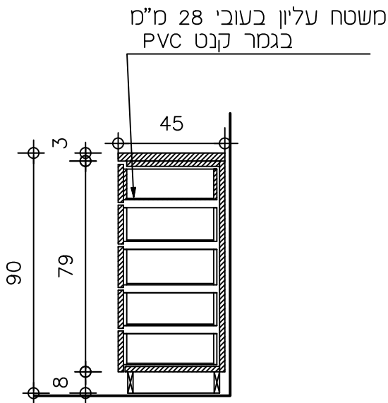
חתך 1:20
