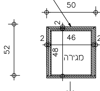
תכנית במגירה 1:20
