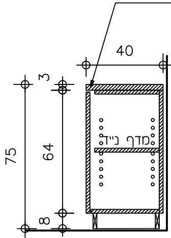
חתך 1:20
