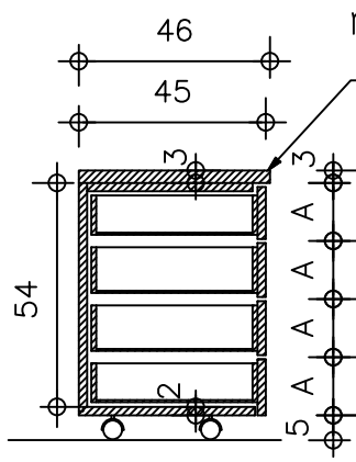
חתך 1:20
