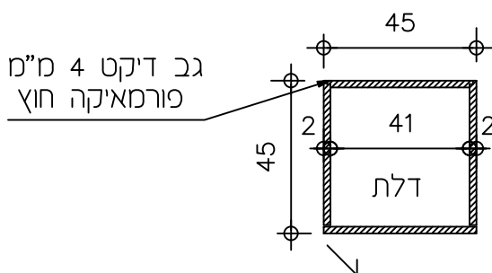
תכנית 1:20
