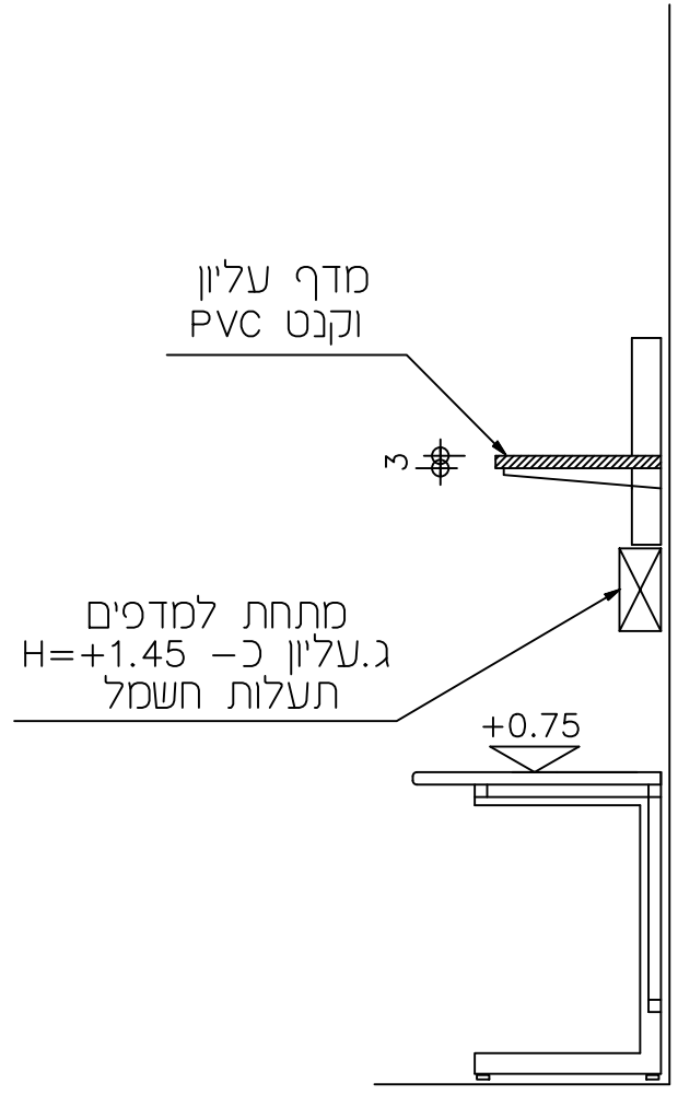
חתך צד 1:20
