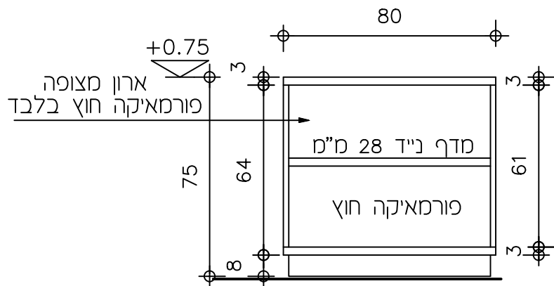
חזית 1:20
