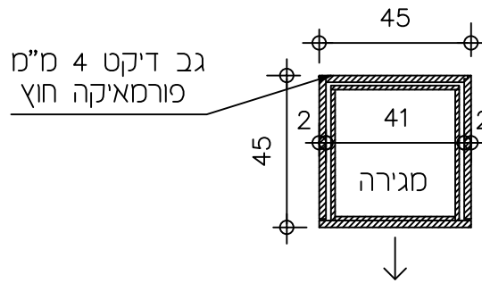
תכנית במגירה 1:20
