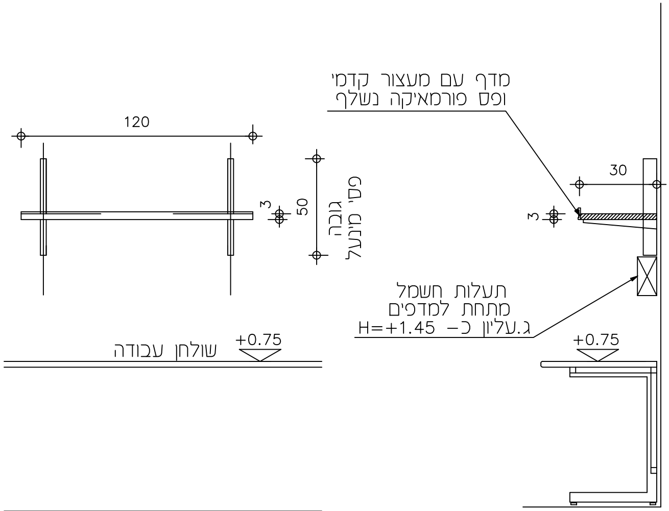
1: 20 מבט
