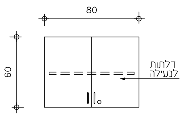
חזית 1:20
