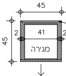
תכנית במגירה 1:20
