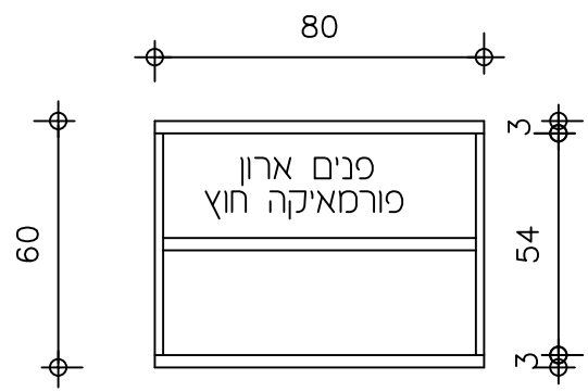
חזית 1:20
