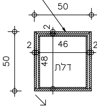
1:20 תכנית בדלת
