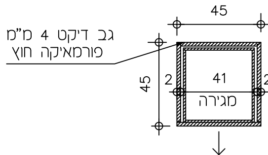
תכנית 1:20
