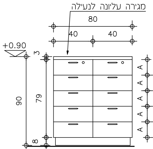
חזית 1:20
