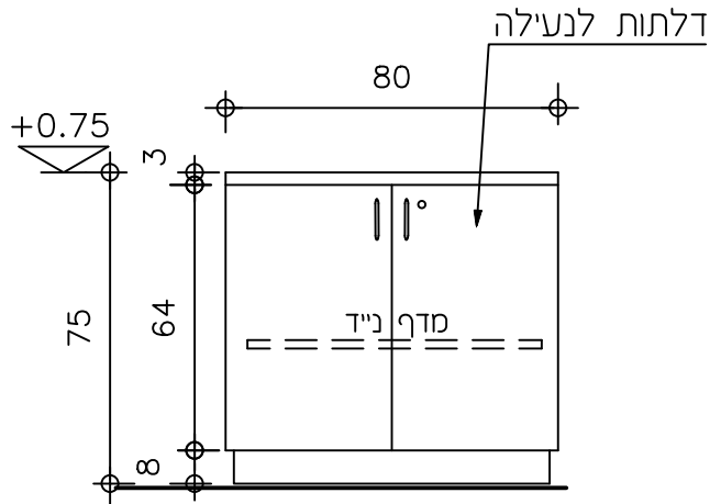
חזית 1:20
