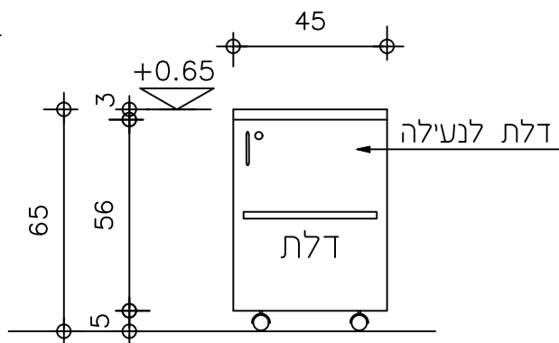
חזית ארונית 1:20
