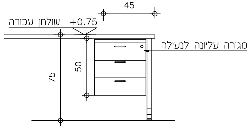
חזית ארונית 1:20
