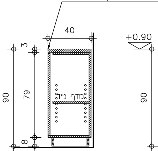
חתך 1:20
