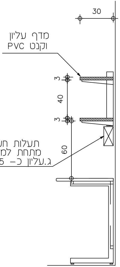
חתך צד 1:20
