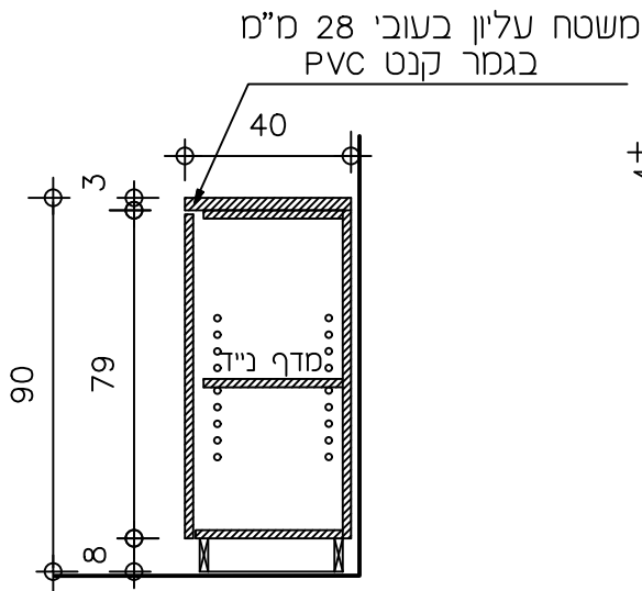
חתך 1:20
