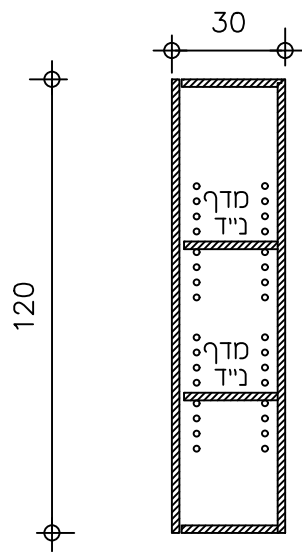
חתך 1:20
