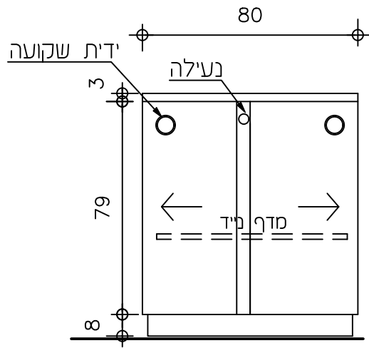
חזית 1:20
