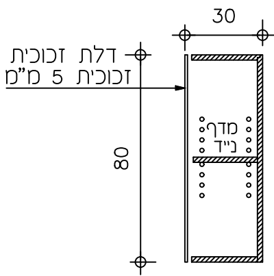
חתך 1:20
