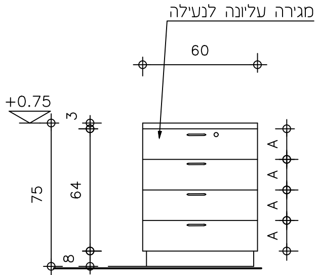
חזית 1:20
