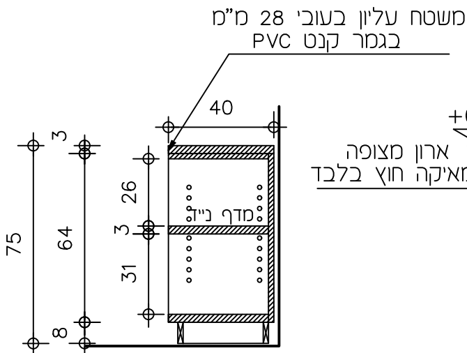
חתך 1:20
