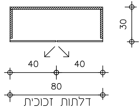
תכנית ארון 1:20
