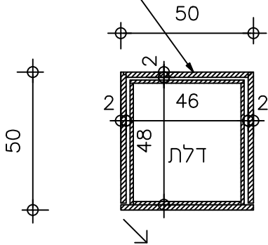
תכנית בדלת 1:20
