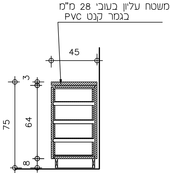
חתך 1:20
