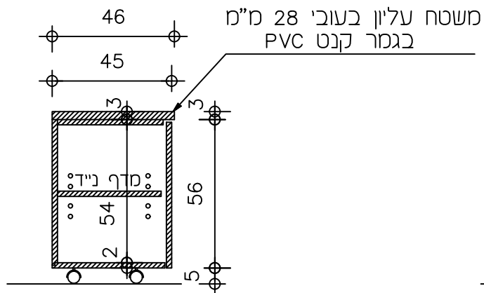
חתך 1:20
