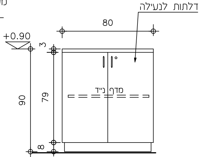
חזית 1:20
