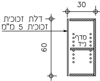
חתך 1:20
