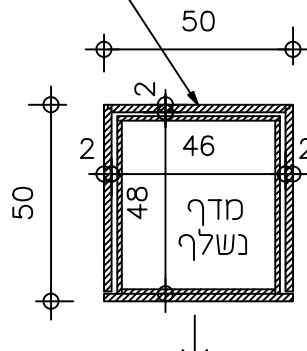
1:20 תכנית במגירה
