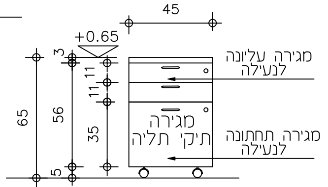
חזית ארונית 1:20
