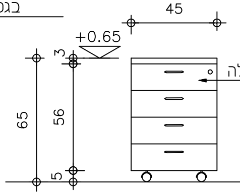
חזית ארונית 1:20
