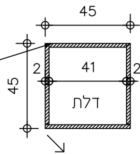
תכנית בדלת 1:20
